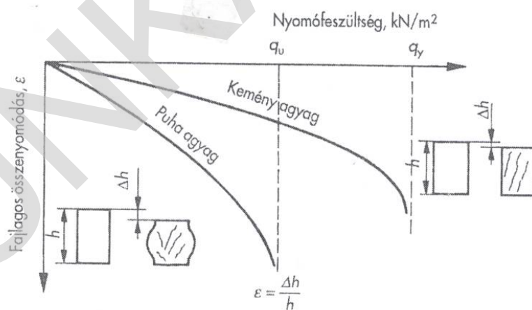
A puha és kemény agyag alakváltozási görbéi az egyirányú nyomóvizsgálat során
