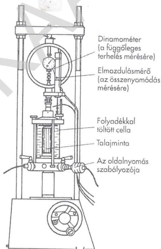
Háromtengelyű triaxális nyomókészülék elrendezési rajza 4
