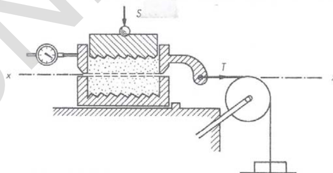
A talajok közvetlen nyírására használt készülék és működése 2
