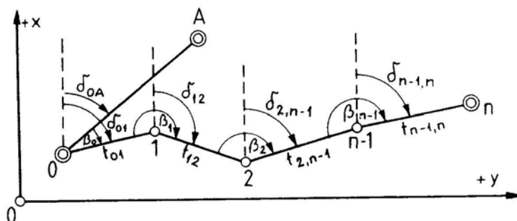
14. ábra. Tájékozott és ismert alappontban végződő sokszögvonal 14
