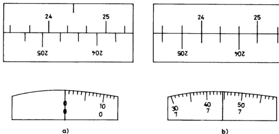
4. ábra. Koincidenziás leolvasó berendezés, a beállítás előtt előtt;b) koincidenzia után leolvasás 24^{\circ}27'44,6''
