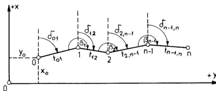
12. ábra. Önálló sokszögvonala 12
