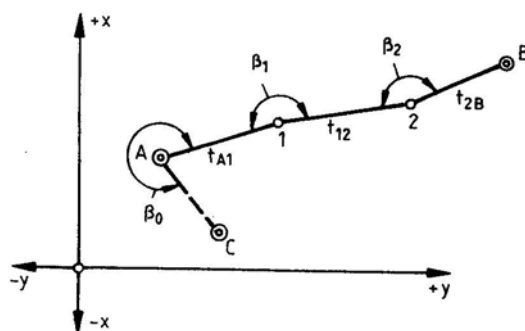
20. ábra. Egyszeresen tájékozott sokszögvonal számítása 20
