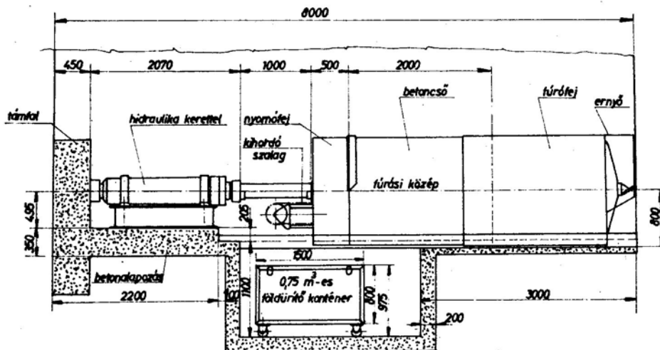
27. ábra. Csőátsajtoló berendezés 27
