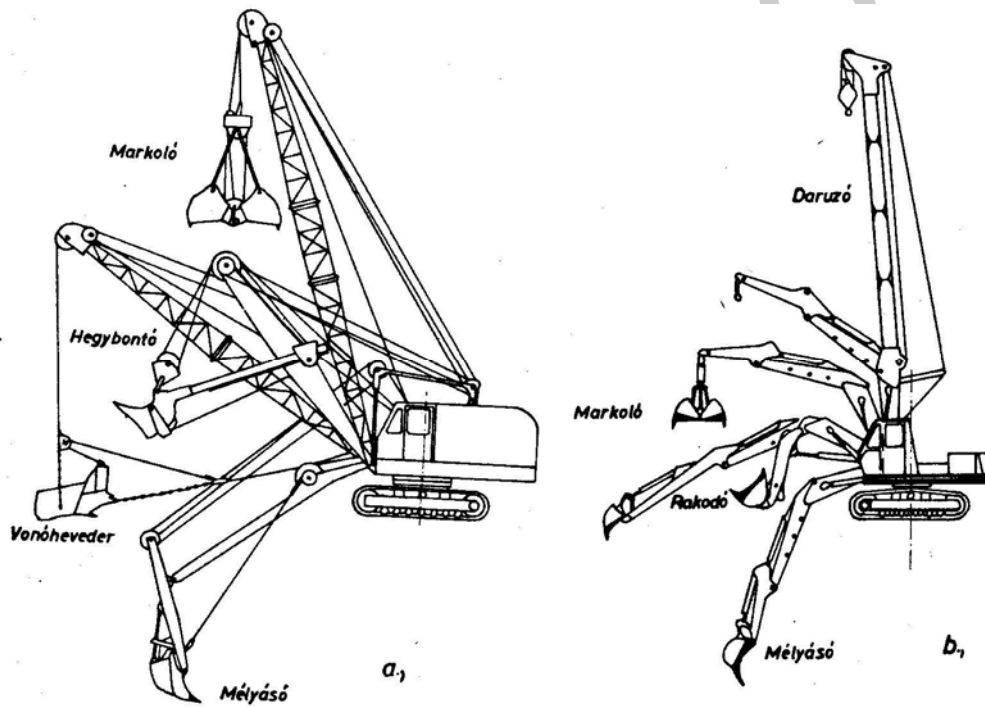
5. ábra. Kotrógépek munkaeszközei 5
