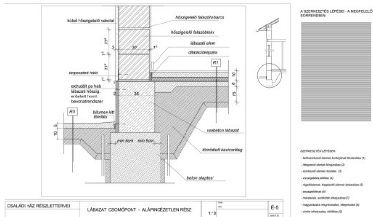
8. ábra csomópontok 1
