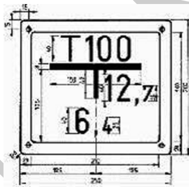
27. ábra. Tűzcsapot jelző tábla
