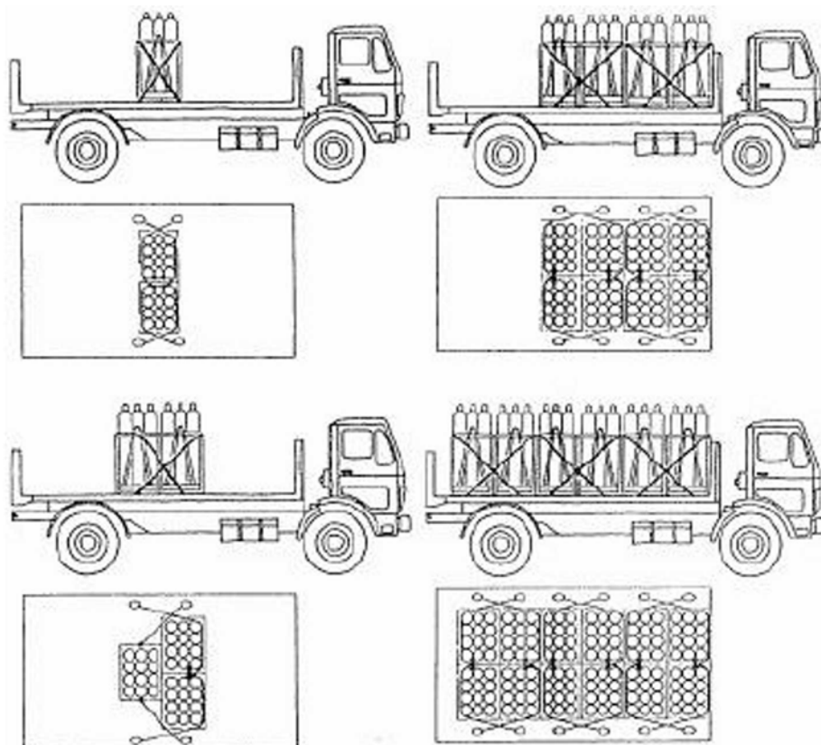
18. ábra. Palackok szállítása
