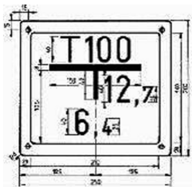
32. ábra. A tűzcsapot jelző tábla vázlata
