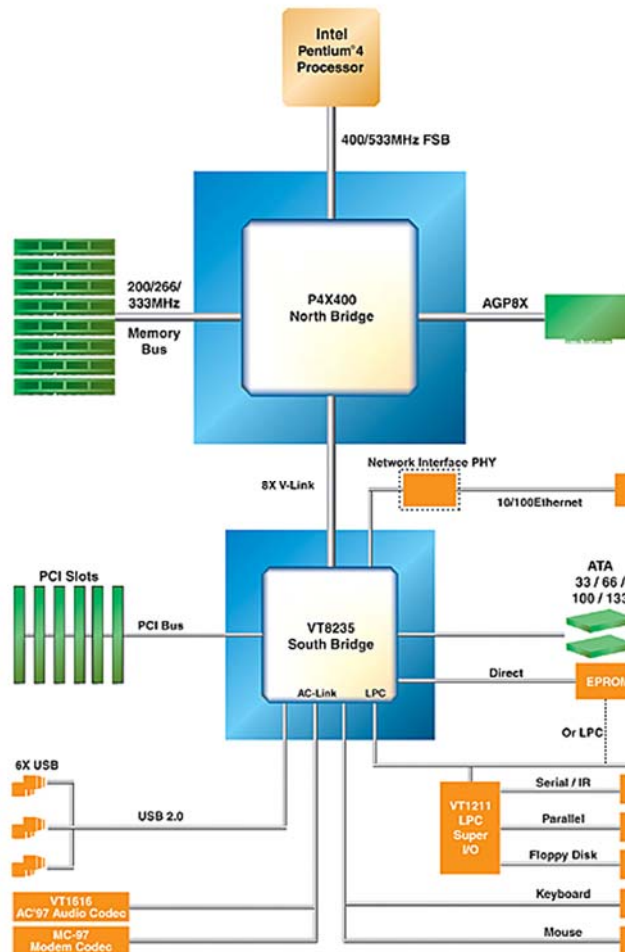
12. ábra. Alaplapi eszközök kapcsolata
