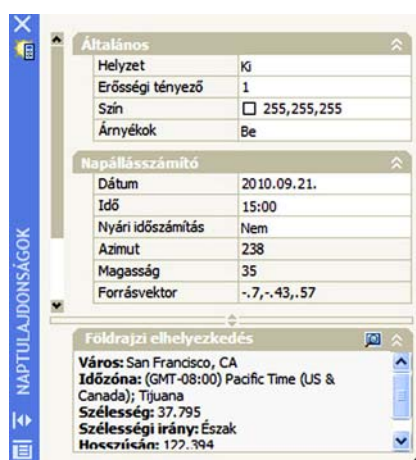
8. ábra. Napállásszámító
