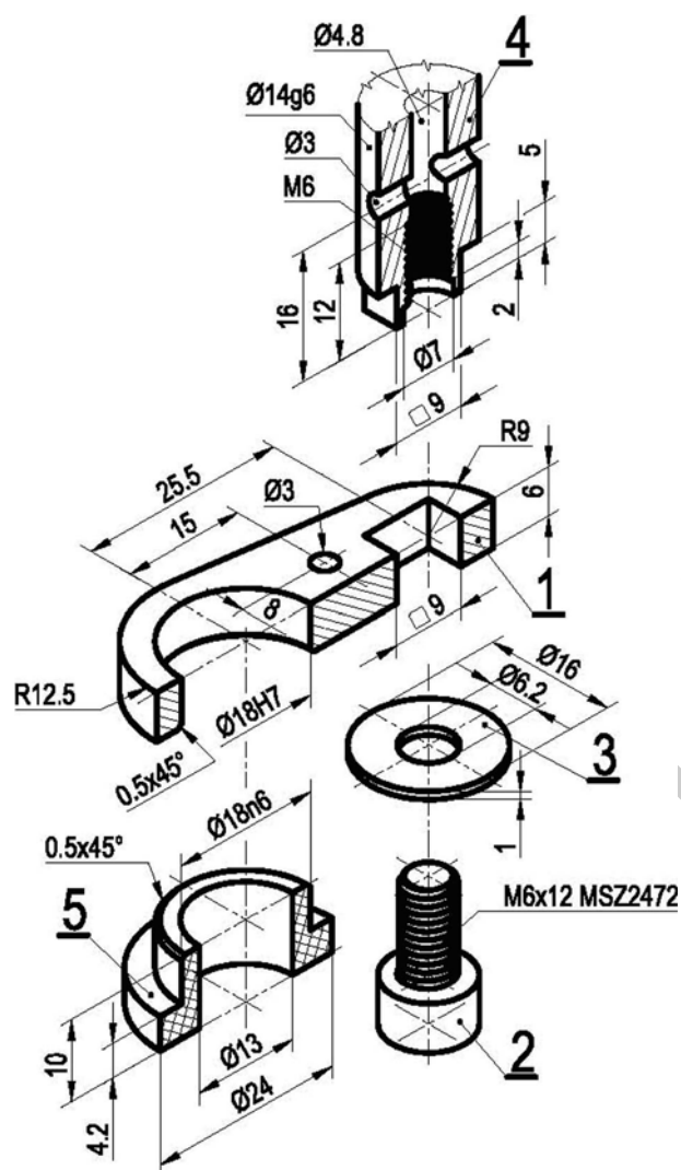
36. ábra. Robbantott ábra
