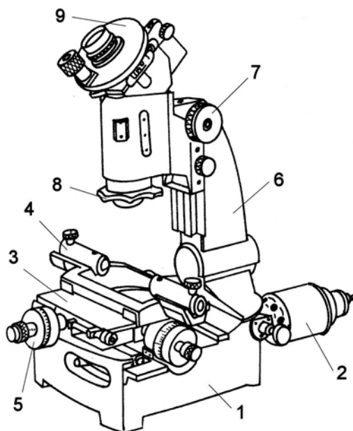
3. ábra. Műhelymikroszkóp 3
