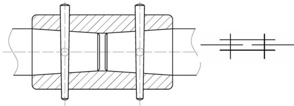
3. ábra. Tokos tengelykapcsoló metszeti és jelképi rajza
