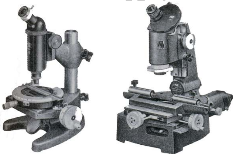
6. ábra. Műhelymikroszkópok 6
