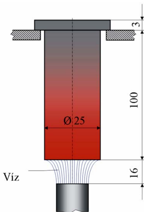
29. ábra. Jominy-féle véglapedzés
