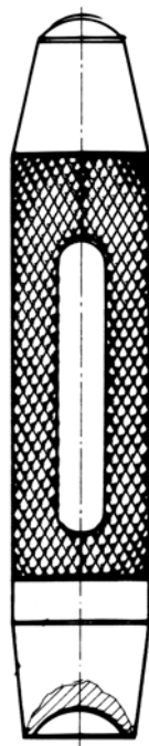
16. ábra. Szegecsfejező
