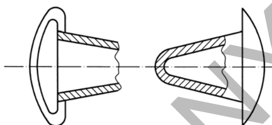
25. ábra. Kétrészes csőszegecs rajza
