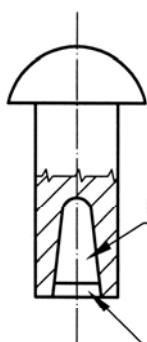
Robbanószegecs
