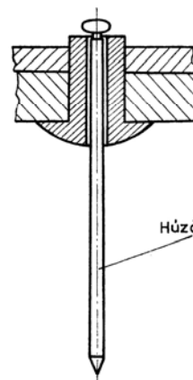
Húzószegecs (POP)
