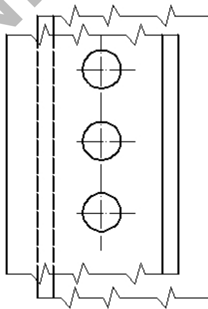
10. ábra. Egysoros átlapolt szegecskötés
