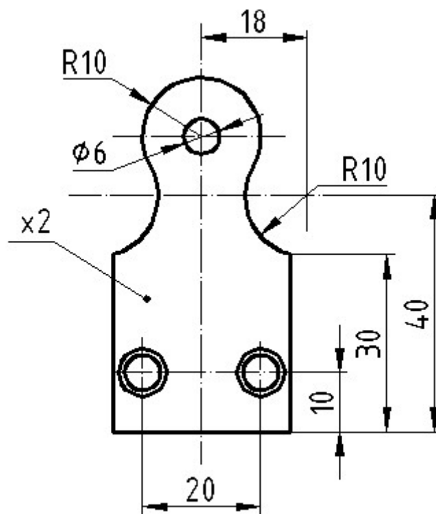
20. ábra. Feladatrajz
