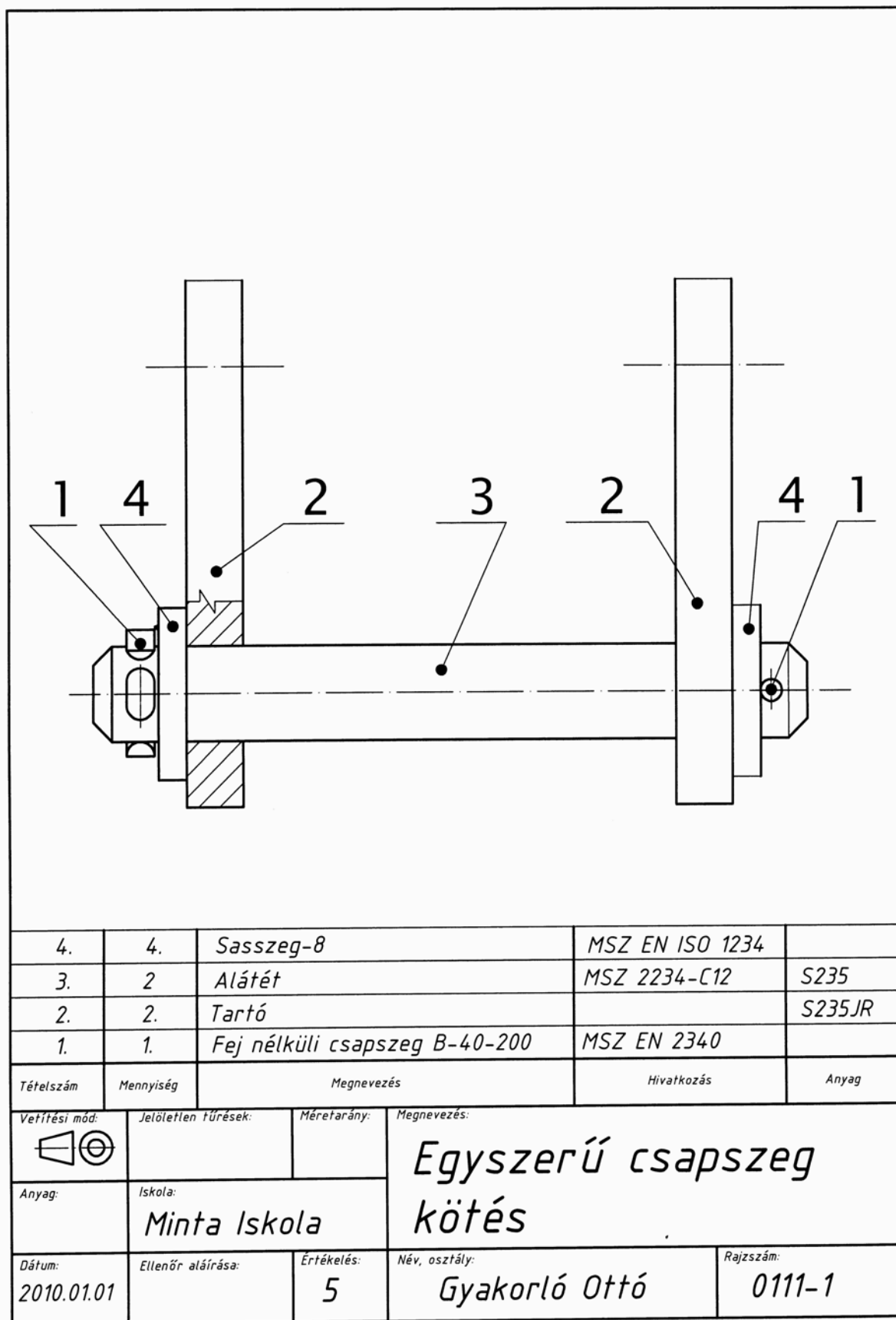
4. ábra. Feliratmező és darabjegyzék
