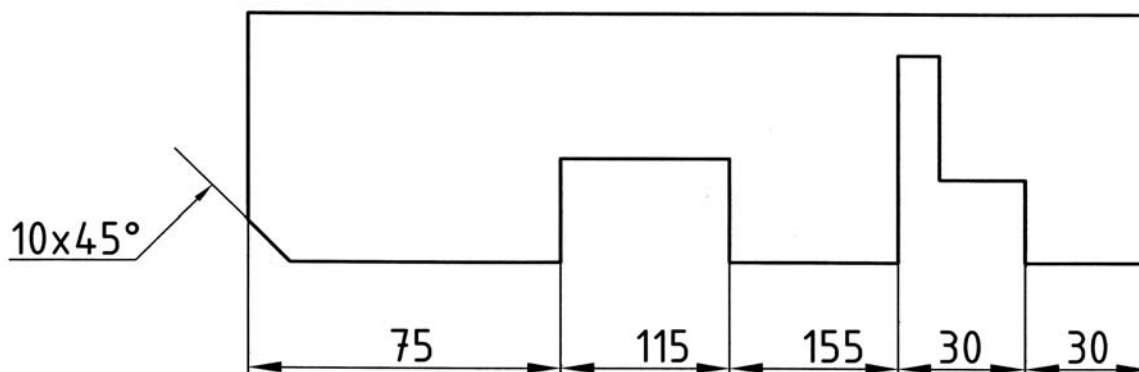
9. ábra. Láncméretezés
