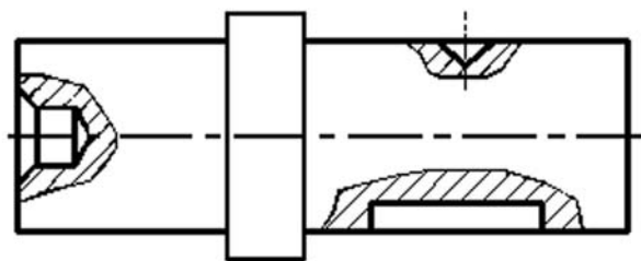
16. ábra. Kitöréses metszet
