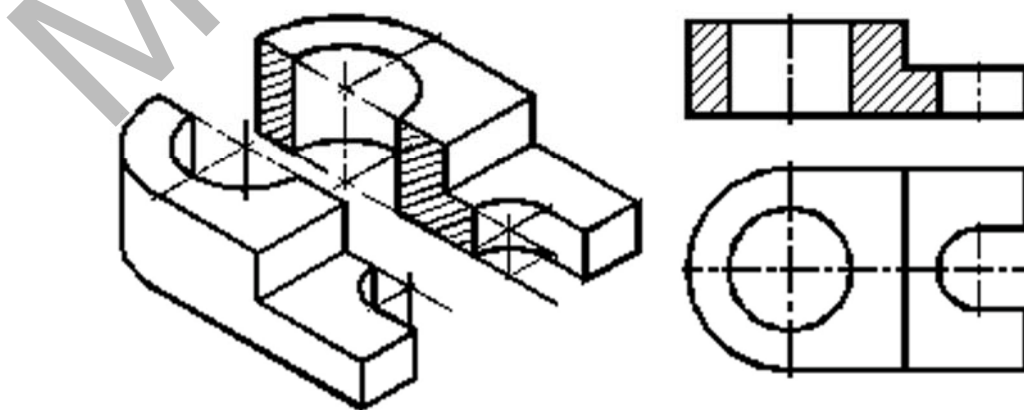
13. ábra. Teljes metszet
