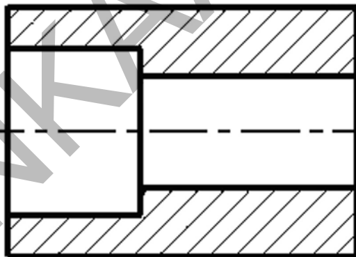
6. ábra. Metszeti vonalkázás
