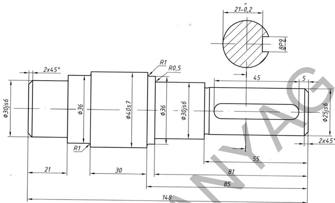
23. ábra. Szelvény alkalmazása nézeten kívülre rajzolva
