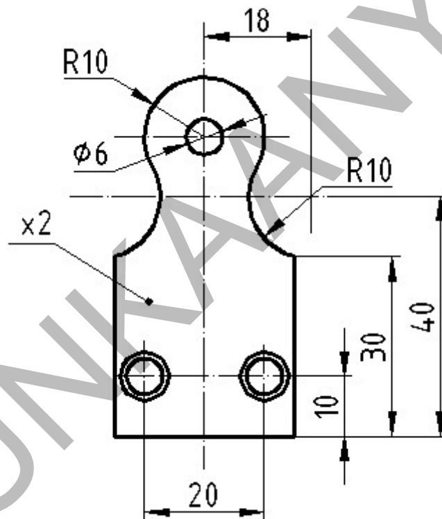
1. ábra Lemeztárgy rajza
