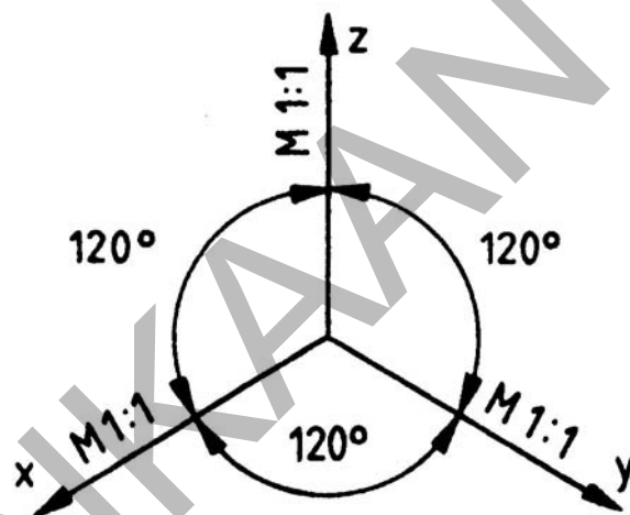
10. ábra. Egyméretű axonometrikus ábrázolás
