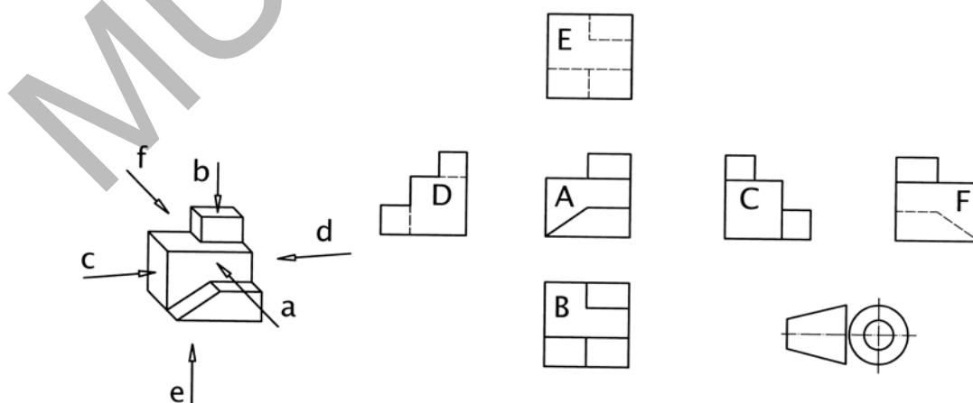
5. ábra. A nézetek képzési irányának jelölése. Európai nézetrend
