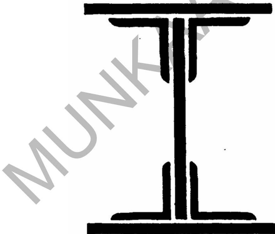
16. ábra. Kis keresztmetszetű rajz metszeti ábrázolása
