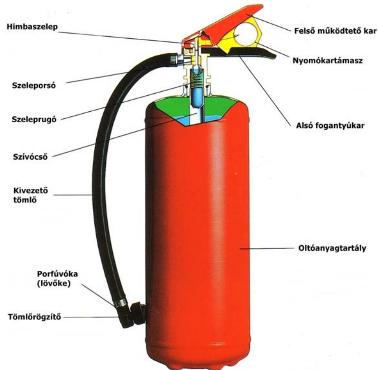
36. ábra. Porraloltó készülék szerkezeti felépítése 36
