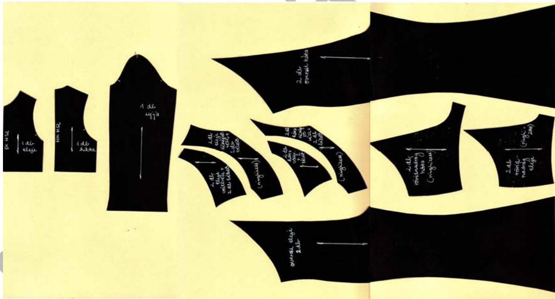
37. ábra. Az előző ábrán szereplő divatgrafikához tartozó méretarányosan lekicsinyített szabásminta
