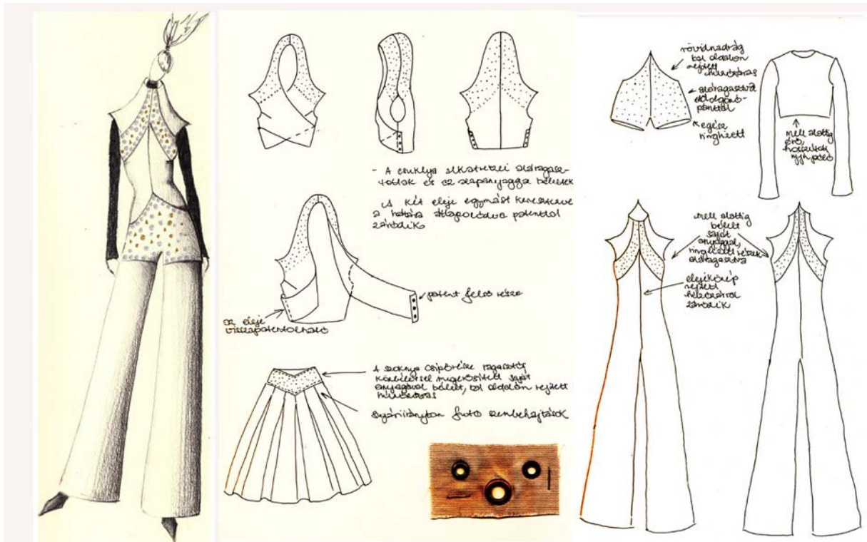
36. ábra. Divatgrafika, műhelyrajz, kellék minta
