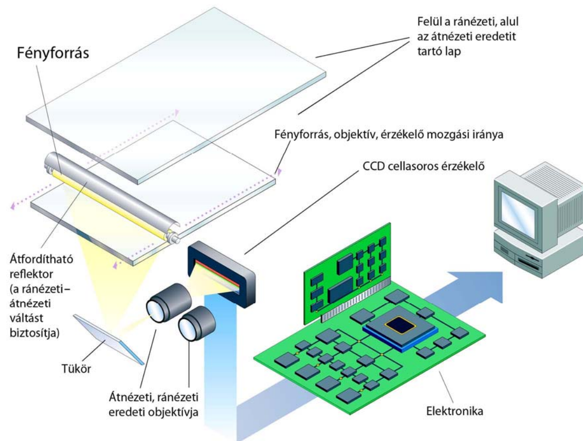
7. ábra. Egy professzionális szkennerek felépítése. Az együtt mozgó fényforrásból, tükörből, objektívokból, CCD-cellából álló letapogató rendszer most éppen átnézeti eredetiről juttatja az információt az elektronikának
