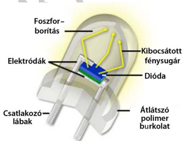
5. ábra. A fehérfényű LED-ek felépítése
