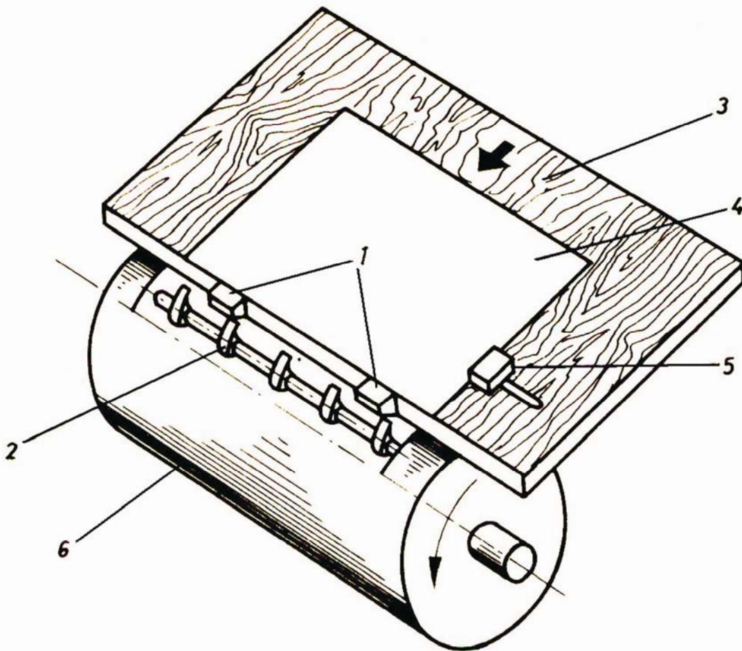
9. ábra. A hárompontos ívillesztés. 1. alapilleszték, 2. ívfogók, 3. ívlevezető asztal, 4. illesztés alatt lévő nyomathordozó, 5. oldalilleszték, 6. ellennyomó henger.
