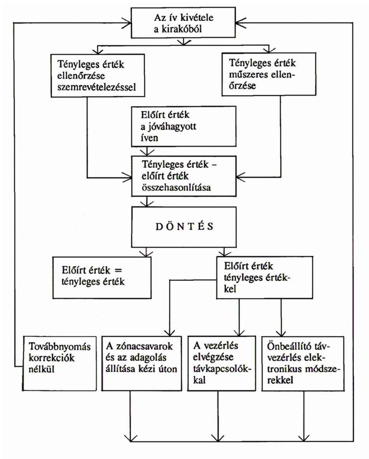
33. ábra. A festékterhelés ellenőrzésének folyamatábrája
