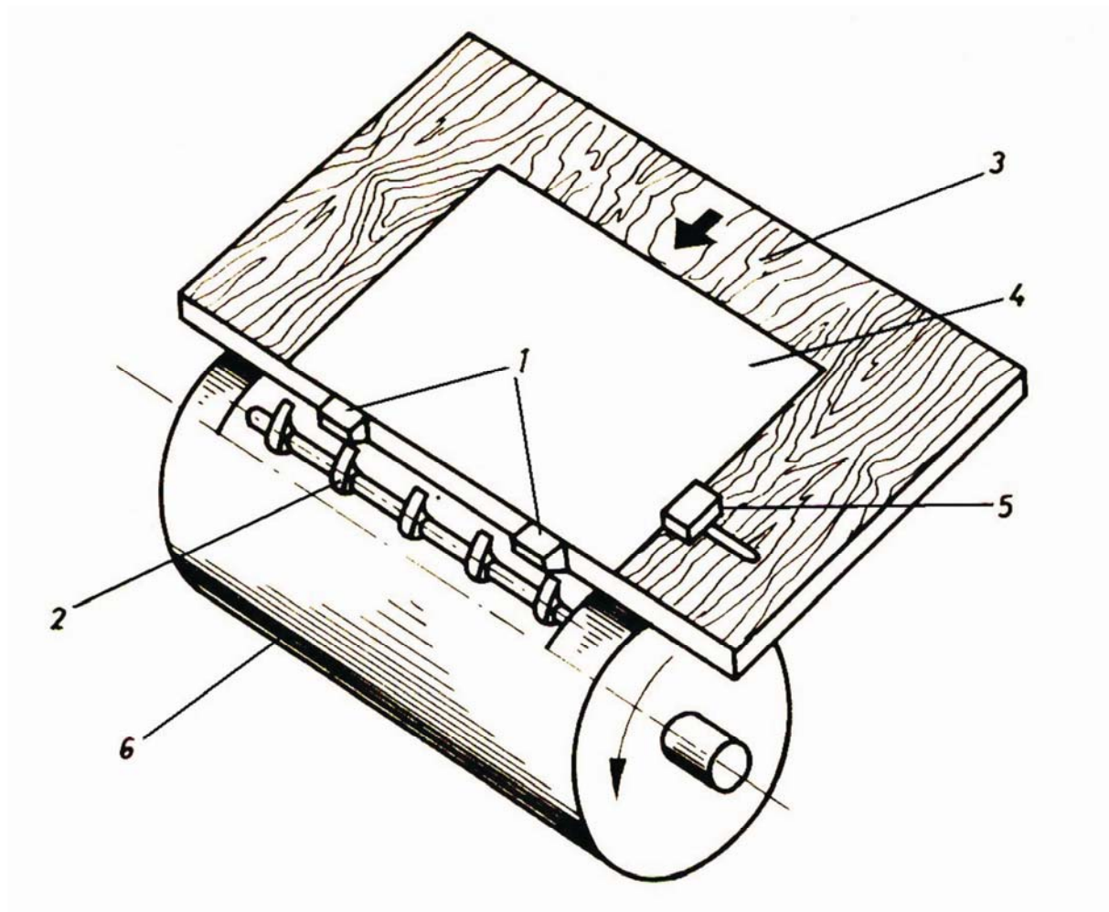
26. ábra. A hárompontos ívillesztés. 1. alapilleszték, 2. ívfogók, 3. ívvezető asztal, 4. illesztés alatt lévő nyomathordozó, 5. oldalilleszték, 6. ellennyomó henger.
