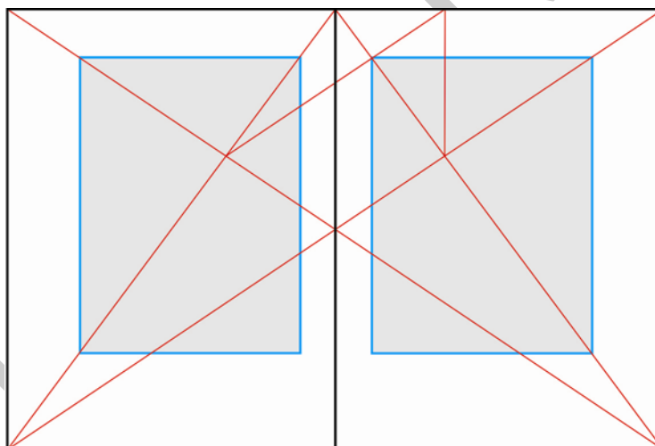
14. ábra. Szedéstükör szerkesztés középkori módszerrel
