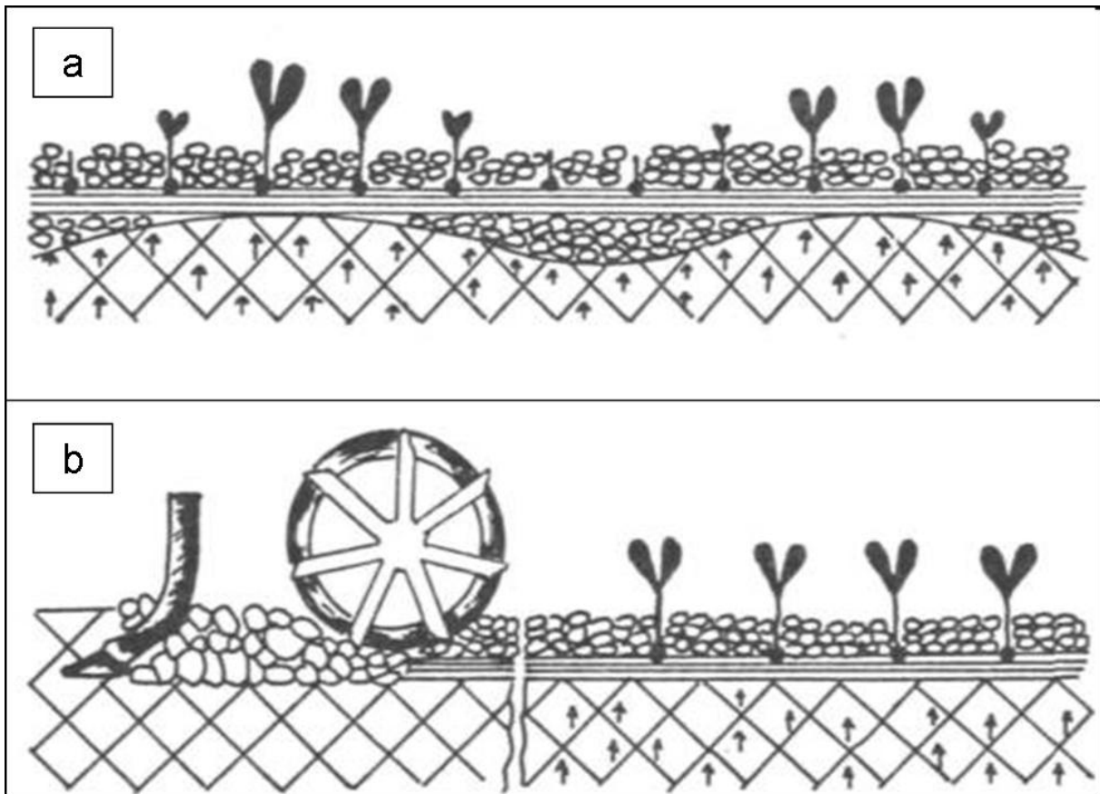
5. ábra. Egyenetlen magágy mélység és kelés (a) és egyenletes (b).
