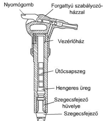
Pneumatikus szegecselőgép
