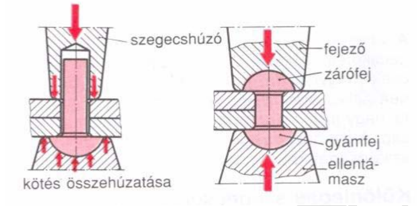
Szegecelés munkafolyamata
