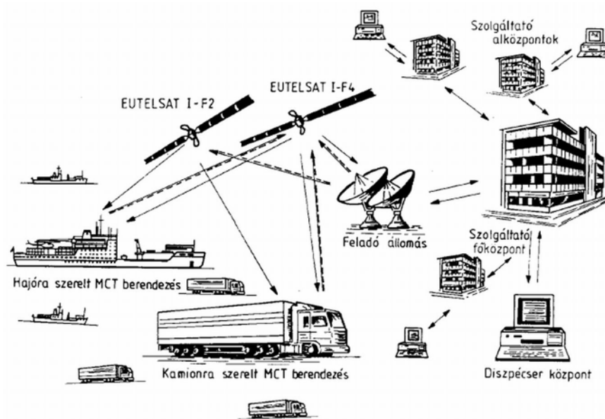
19. ábra. Az EUTELTRACS felépítése 34
