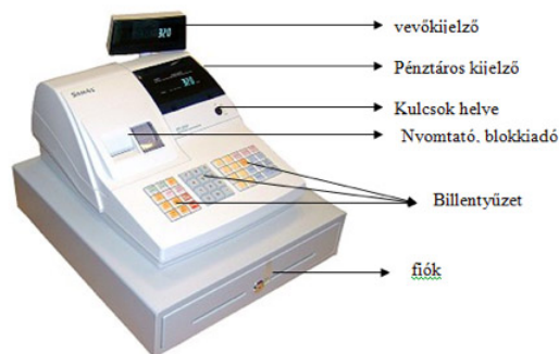
9. ábra elektronikus pénztárgép részei
