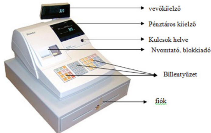
11. ábra elektronikus pénztárgép részei
