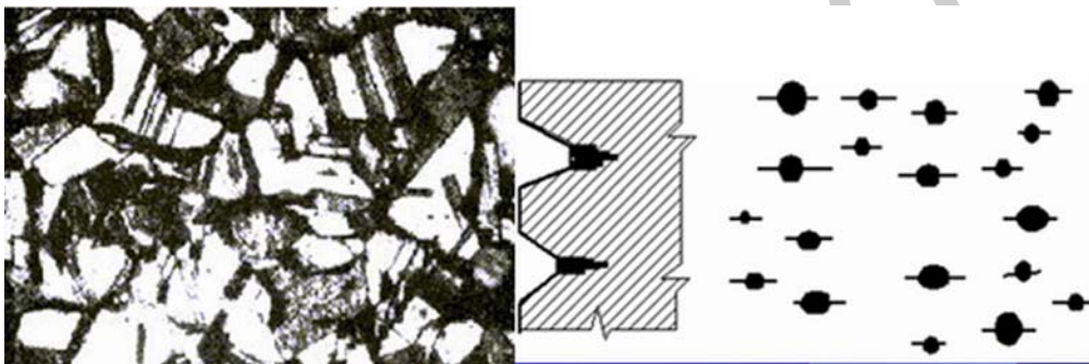
7. ábra. Feszültségi korrózió és korróziós kifáradás
