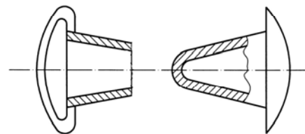
Kétrészes szegecs
