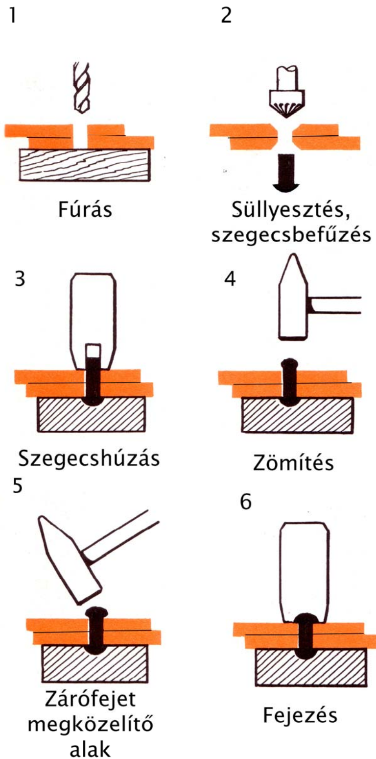
21. ábra. Hagyományos szegecskötés
