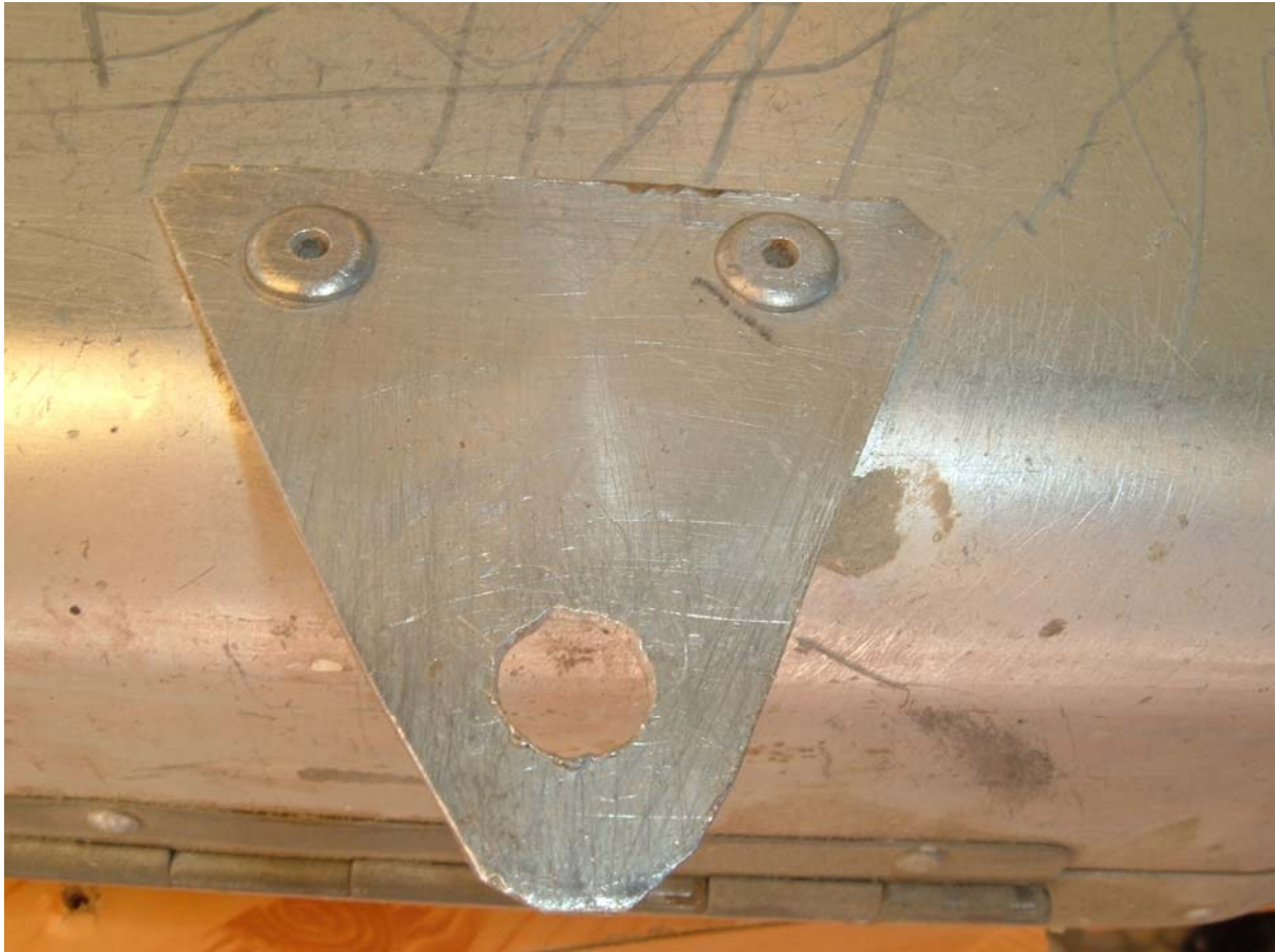
34. ábra. Záró szegecs (POP szegecs) képe a szerelés oldaláról
