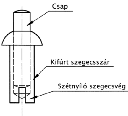
Csapos szegecs
