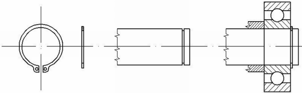
15. ábra. Rögzítő gyűrű beépítése tengelyre
