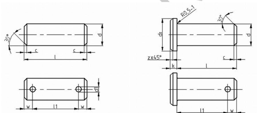
6. ábra. Menetnélküli csapszegek táblázathoz
