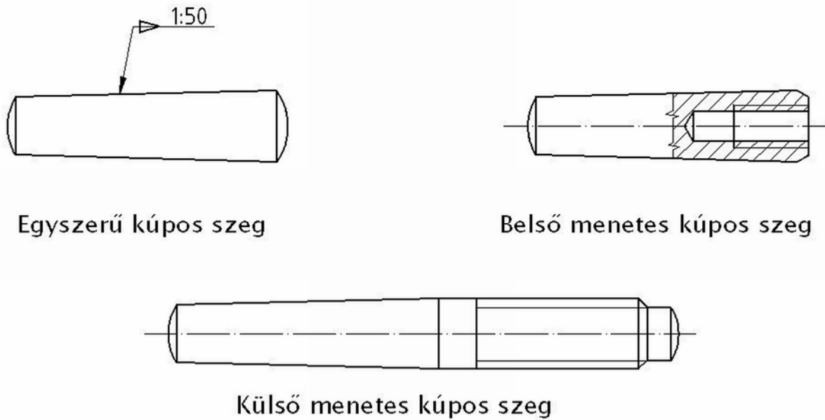
30. ábra. Kúpos szegek
