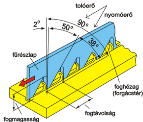
15. ábra fűrészlap forgács leválasztása
