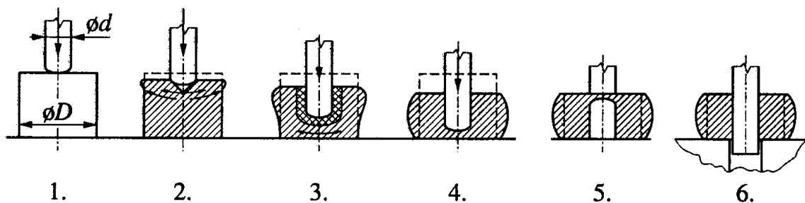
7. ábra. A kovácslyukasztás folyamata
