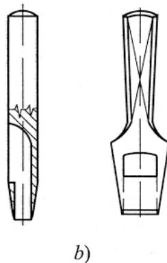
9. ábra. Bőrlyukasztók a) egyszerű; b) kengyeles
