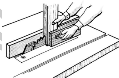
32. ábra. Csap befűrészélése asztalos körfűrészgépen
