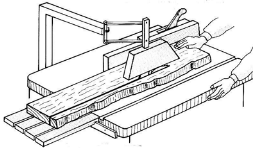
28. ábra. Hasítás asztalos körfűrészgépen
