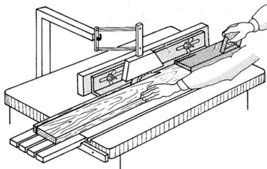
30. ábra. Lécvágás pótvezetővel és tolódeszkával
