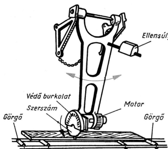
1. ábra. Ingafűrészgép
