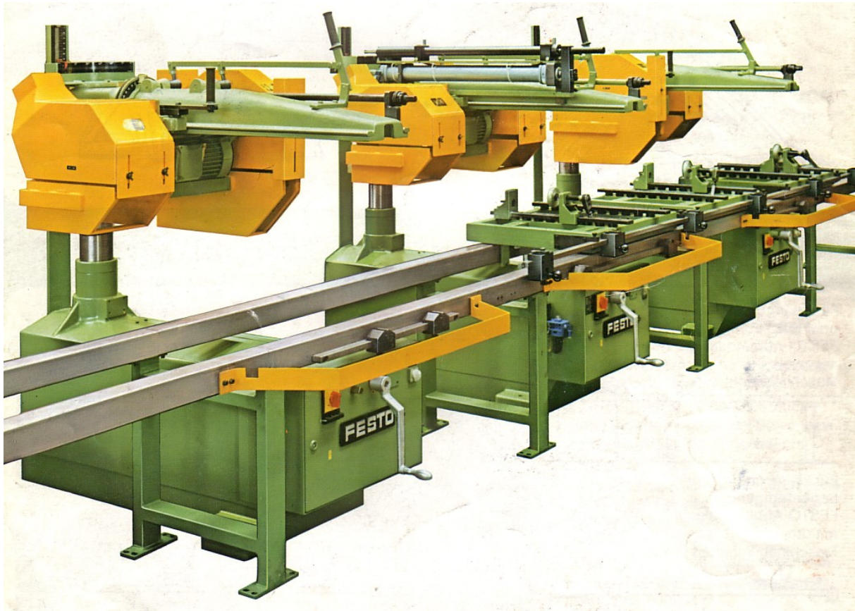
2. ábra. Karos leszáró körfűrészgép 1
