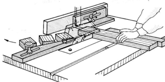
31. ábra. Rövid tuskók vágása
