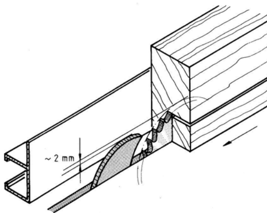
9. ábra. Aljázáskor a hasítóék helyzete
