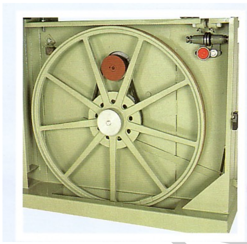
23. ábra. Ékszíjhajtás 8
