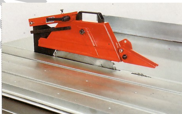
11. ábra. Párhuzam védősisak 4
