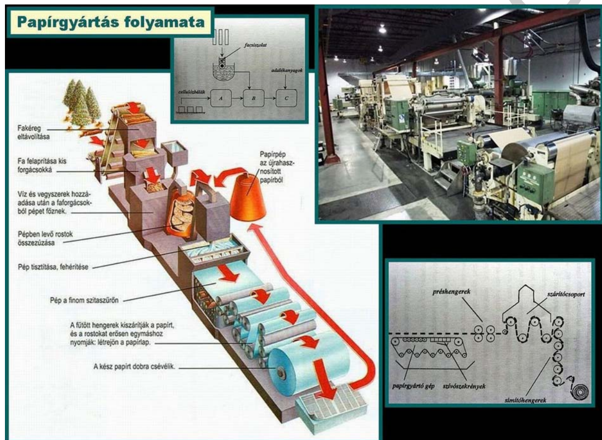
30. ábra. Papírgyártás menete
