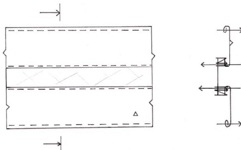
17. ábra. Közepén csipkével díszített futó nézeti és metszeti képe 18
