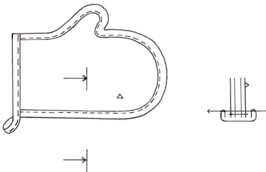
44. ábra. Edényfogó kesztyű rolni pánttal 45
