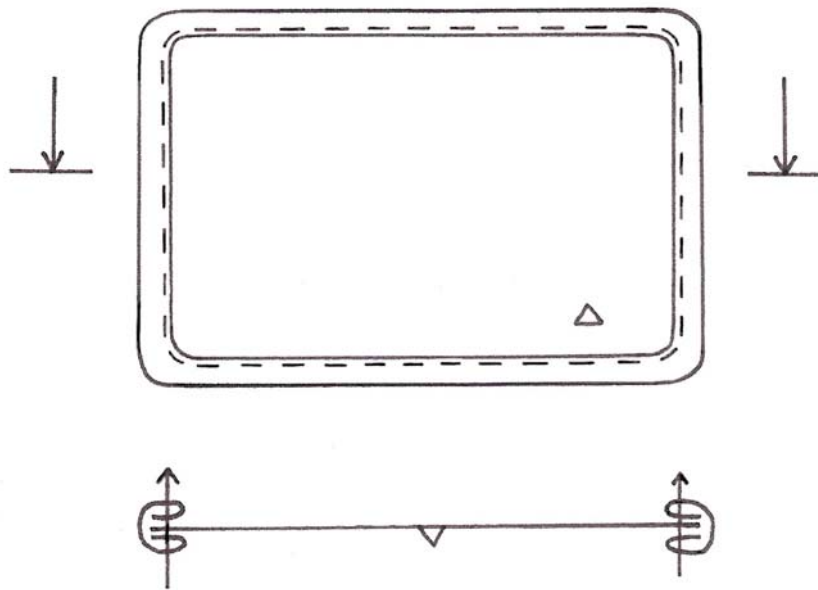
28. ábra. Rolni pántos tányéralátét nézeti és metszeti képe 29
