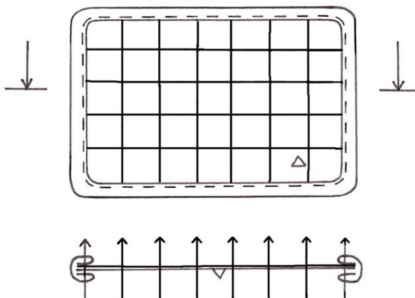
31. ábra. Steppelt rolni pántos tányéralátét nézeti és metszeti képe 32
