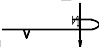
8. ábra. Szegett szövetszélek egyszeres visszahajtása
