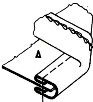
11. ábra. Szegés hajtogató készülék alkalmazásával, szalaggal és ferdepánttal 6
