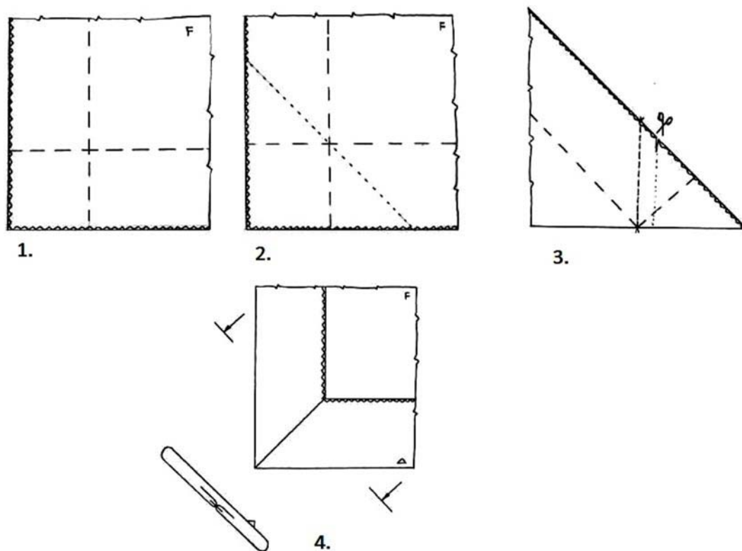
12. ábra. Sarokvarrás készítése 7
