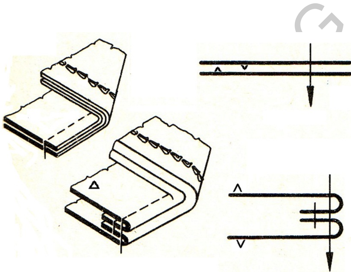
1. ábra. Összevarrás egysoros varrattal 1
