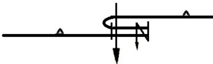
7. ábra. Áttűzéssel megerősített összevarrás
