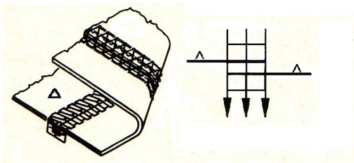
8. ábra. Félbehajtott pánttal történő összevarrás
