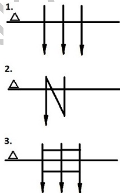
27. ábra. Díszítés különböző varratokkal
