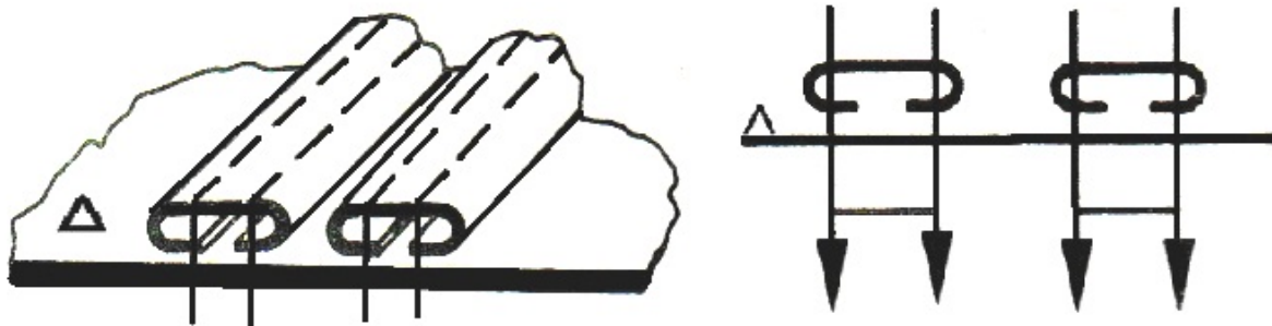
13. ábra. Sportruházatra díszcsíkok felvarrása 9
