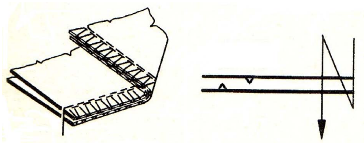
2. ábra. Összevarrás szegővarrattal 2
