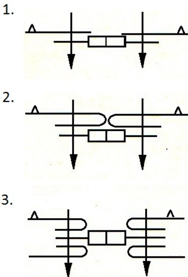
39. ábra. Húzózár bevarrások
