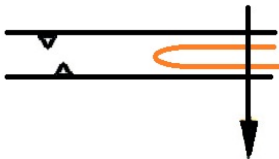
9. ábra. Alul– felülfedő varrattal készült összevarrás 5
