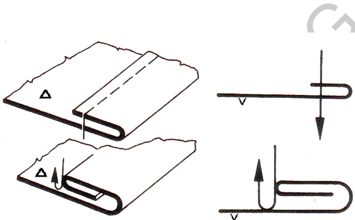
22. ábra. Kelmék szélének elszegése visszahajtással, átmenő és rejtett öltésű varrattal 11
