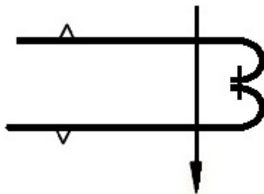
4. ábra. Francia varrás
