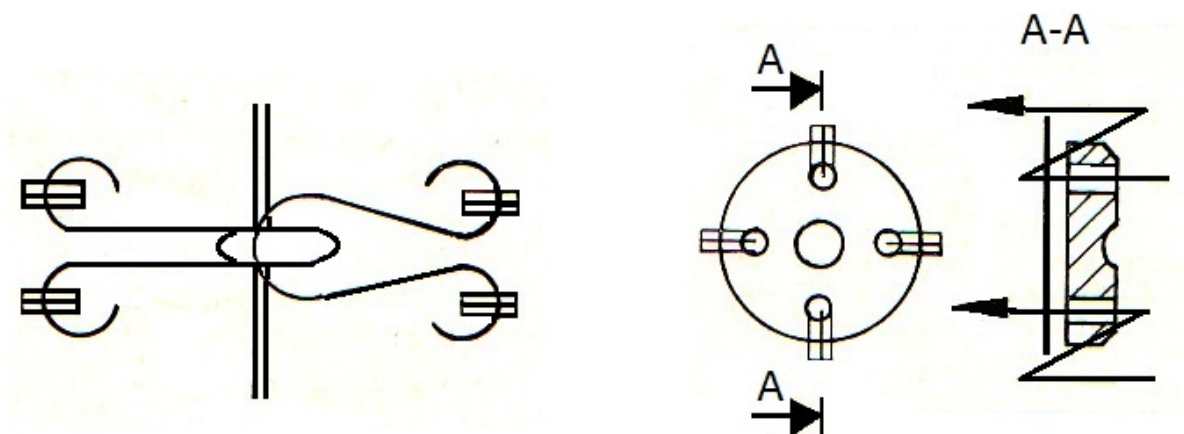
42. ábra. Horgas kapocs és nyomókapocs felvarrása 24
