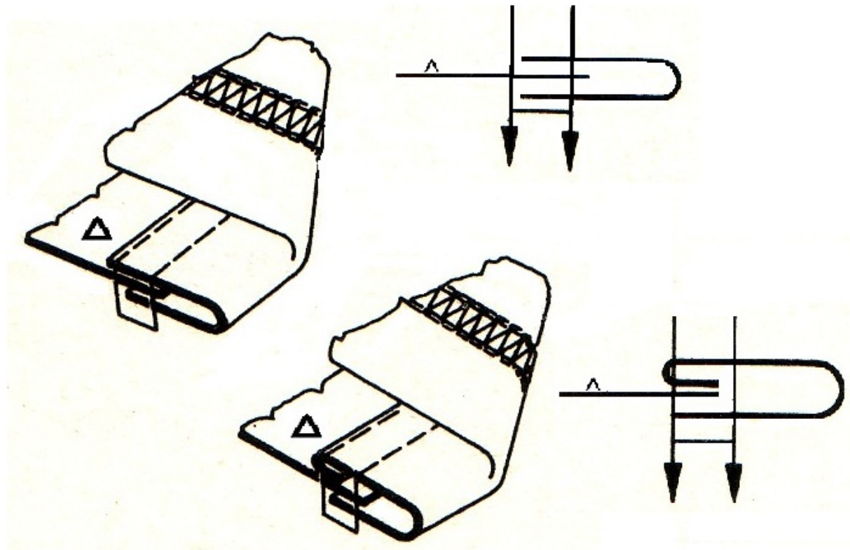
25. ábra. Pántozás fedővarrattal, hajtogató készülék alkalmazásával 13
