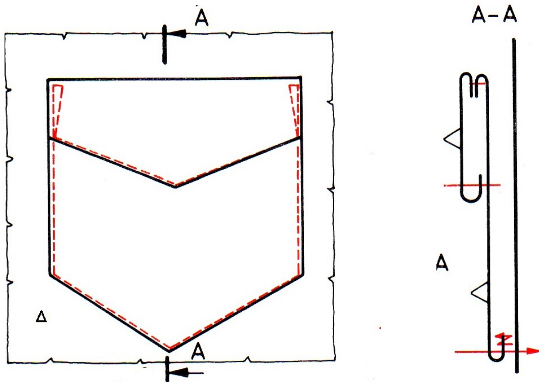
10. ábra. Foltzseb fölvarrása 6
